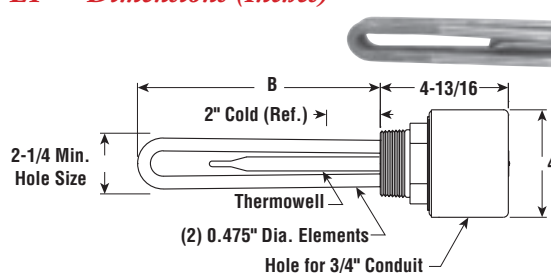
E2 — Dimensions (Inches)
